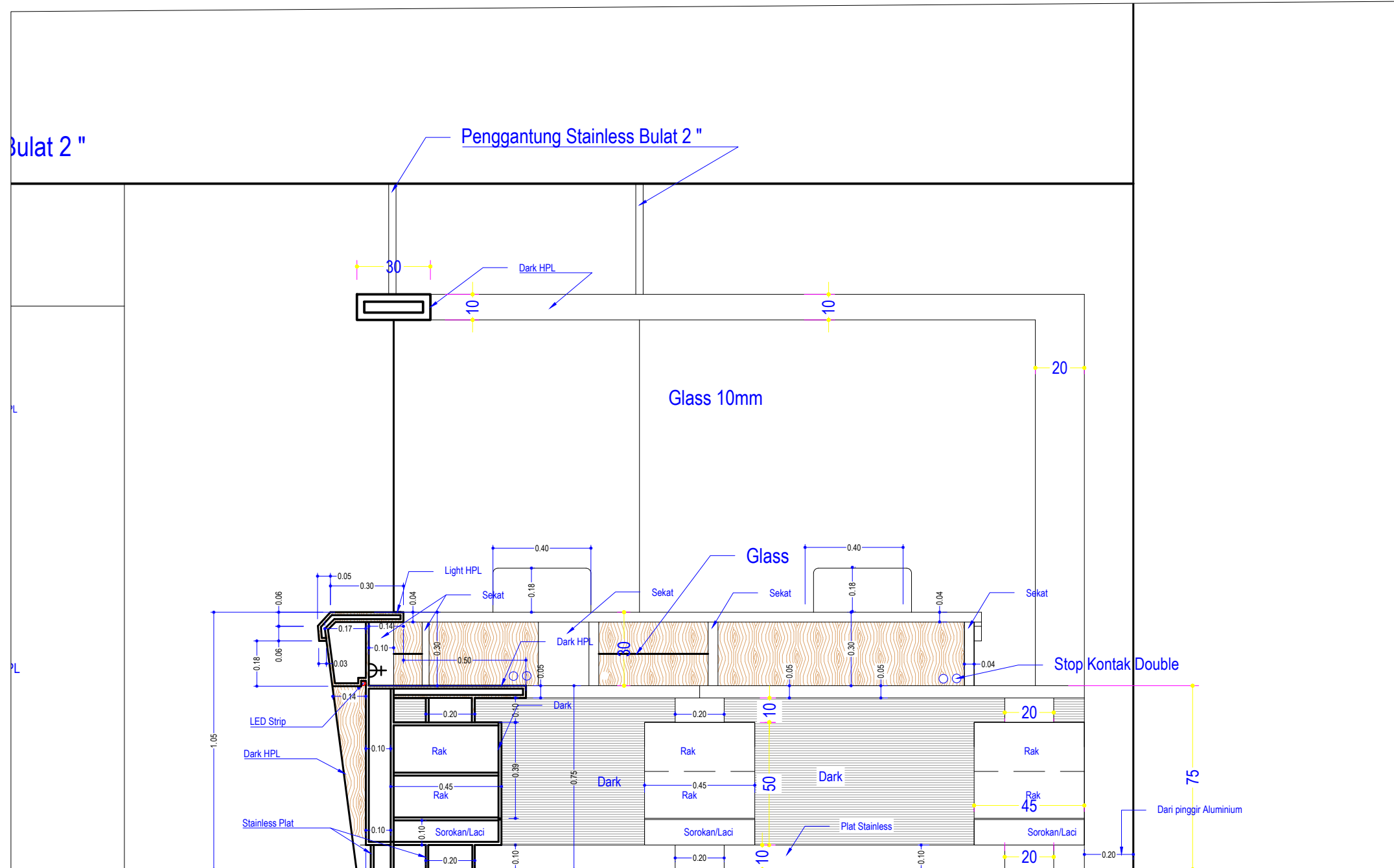
POTONGAN SKALA 1: 10
