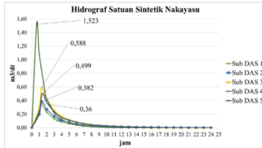
Gambar 5. Kurva HSS Nakayasu Sub DAS Wilayah Studi
