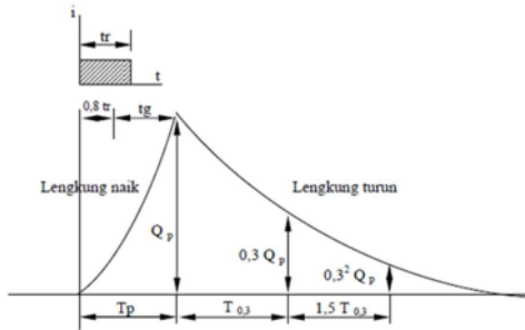
Gambar 2. Hidrograf Satuan Sintesis Metode Nakayasu [18]
