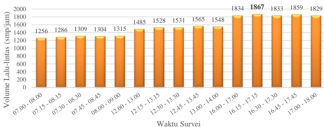
Gambar 7. Penentuan jam puncak di Simpang Waribang
