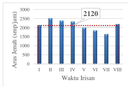
Gambar 8. Diagram arus jenuh pendekat terlindung di Simpang Subita
