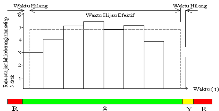
Gambar 2. Pengukuran arus jenuh dengan Metode Time Slice (Sumber: Fadli & Elkhasnet, 2012)
