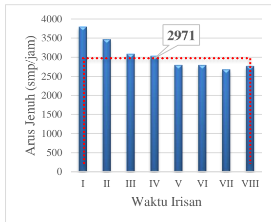
Gambar 11. Diagram arus jenuh pendekatan terlawan di Simpang Waribang
