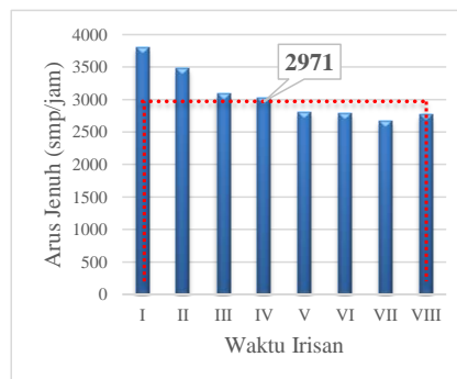
Gambar 9. Diagram arus jenuh pendekat terlawan di Simpang Waribang
