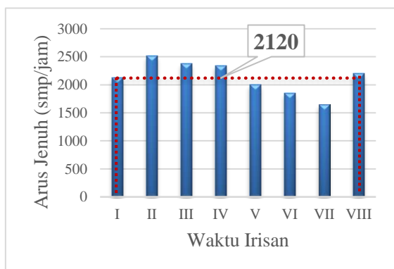
Gambar 10. Diagram arus jenuh pendekatan terlindung di Simpang Subita
