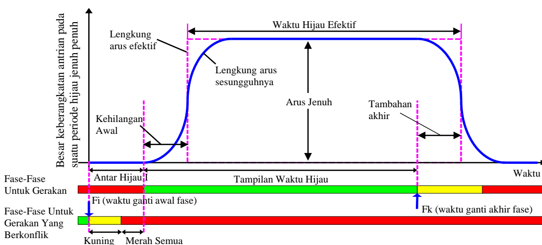
Gambar 1. Model dasar untuk arus jenuh (Sumber: Anonim, 1997)
