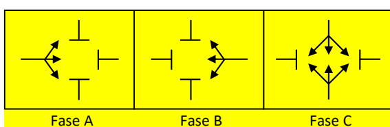
Gambar 8. Diagram fase lalu lintas Simpang Subita
