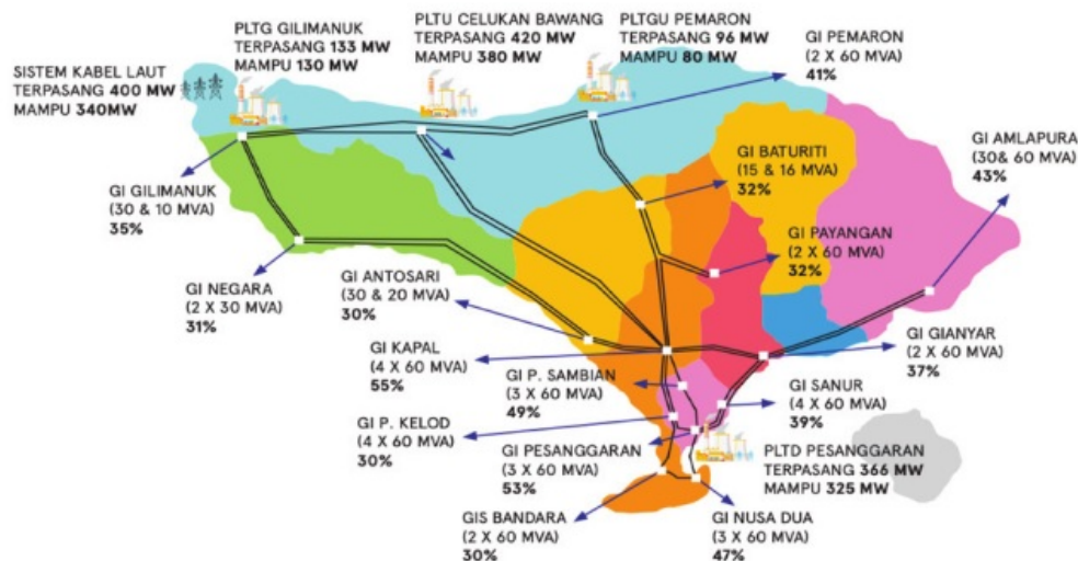
Gambar 8. Sistem kelistrikan Bali
