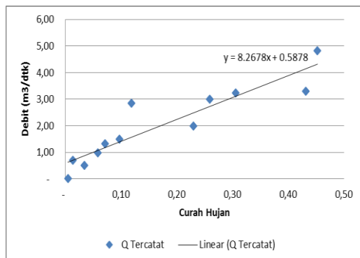
Gambar 5. Hubungan Debit (Q) dan Hujan (P)
