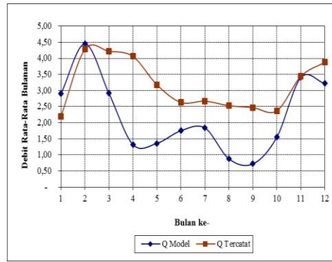
Gambar 7. Debit Limpasan Tahun 1995
