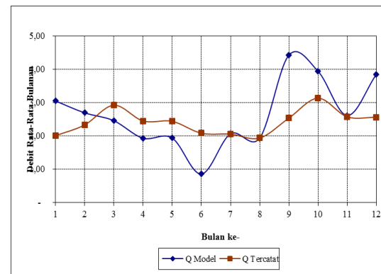
Gambar 10. Debit Limpasan Tahun 1998
