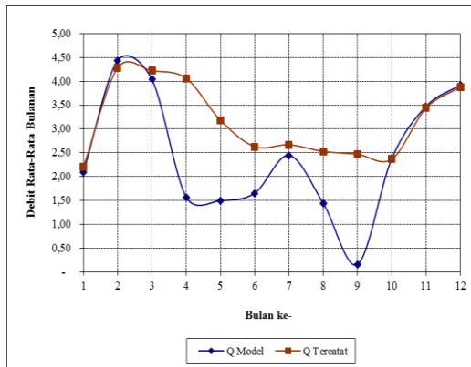
Gambar 12. Debit Limpasan Tahun 1995
