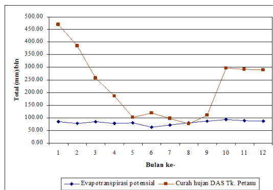
Gambar 4. Curah Hujan Daerah dan Evapotranspirasi
