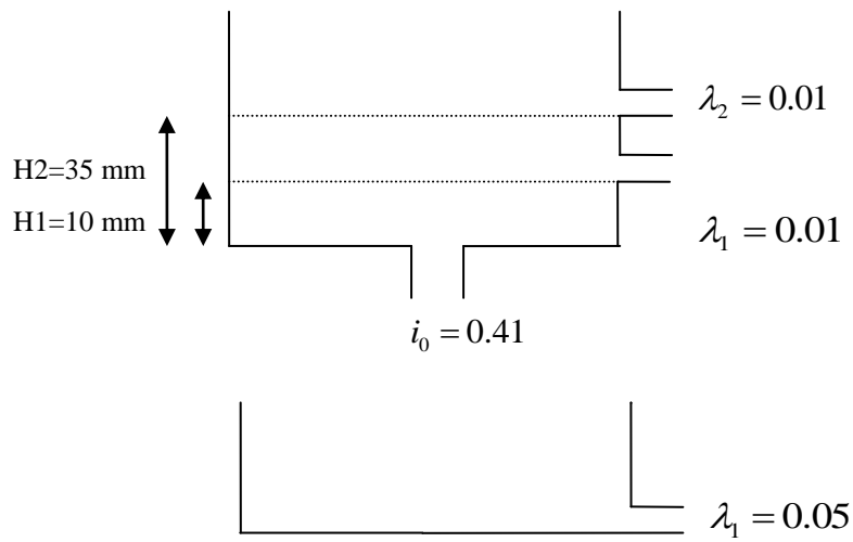
Gambar 12. Susunan Tangki dan Kofesien lubang.
