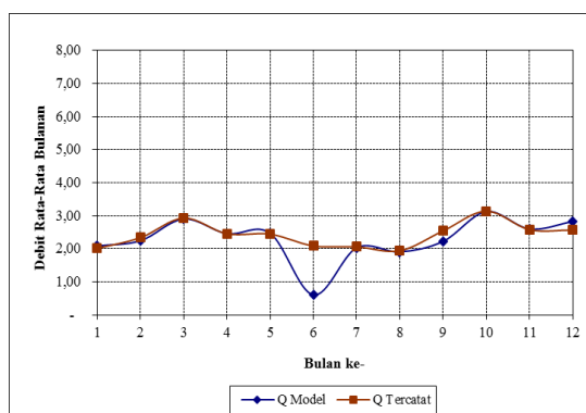
Gambar 15. Debit Limpasan Tahun 1998
