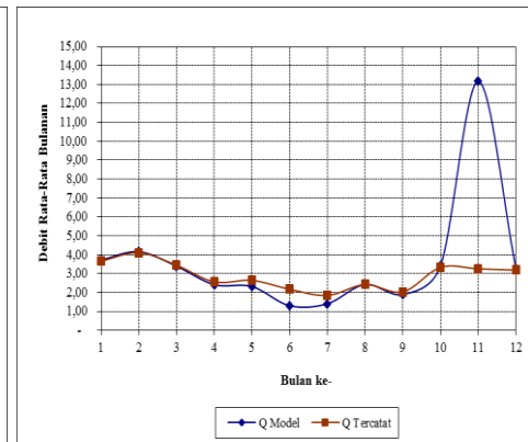
Gambar 13. Debit Limpasan Tahun 1996
