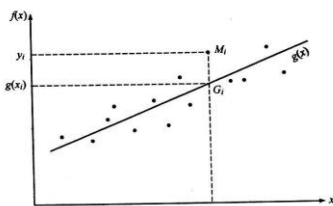
Gambar 1. Sebaran Hidrograf Regresi Linier
