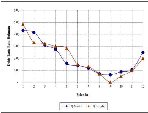
Gambar 6. Debit Limpasan Tahun 1994
