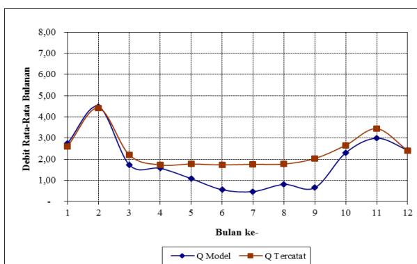
Gambar 14. Debit Limpasan Tahun 1997
