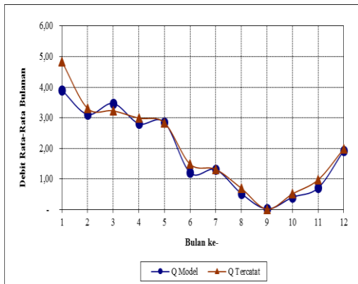
Gambar 11. Debit Limpasan Tahun 1994
