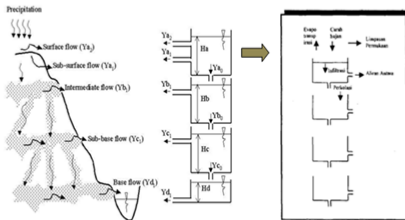
Gambar 1. Konsep Model Tangki Gambar 2. Struktur Model Tangki
