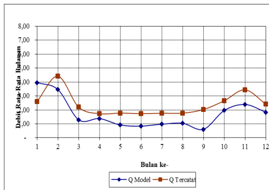
Gambar 9. Debit Limpasan Tahun 1997
